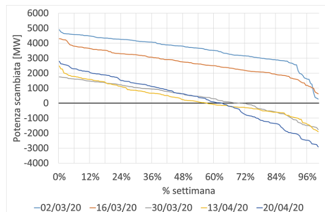
Figura 1.21 – Curva di durata scambio di potenza Italia-Francia nelle settimane indicate (elaborazione ESL@energycenter/Polito su dati Terna)
