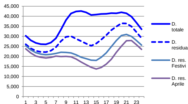
Figura 6.28 – Domanda residua media oraria nei giorni festivi
