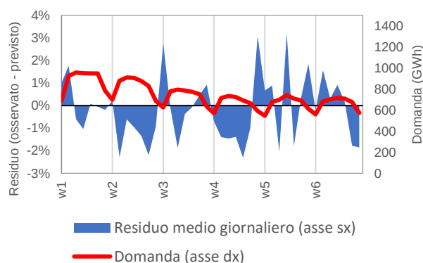
Figura 1.8 – Domanda di energia elettrica (TWh) e indicazione della variazione percentuale rispetto al 2019 tra la prima settimana di marzo (w1) e la seconda settimana di aprile (w6) nel 2020
