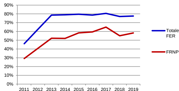
Figura 6.25 – Percentuale di produzione da FRNP nello 0,1% delle ore di massima penetrazione (% sul carico)
