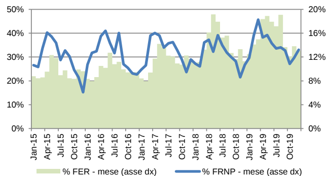
Figura 6.24 – Produzione elettrica da FER e da sole rinnovabili intermittenti (% della richiesta di energia elettrica)
