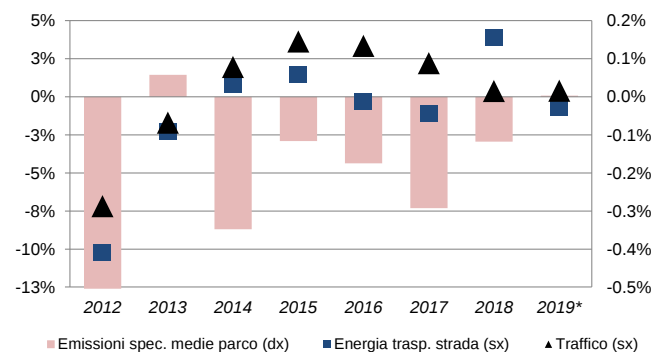
Figura 4.17 – Variazioni annuali % delle emissioni medie di CO 2 /km del parco auto (asse dx), dei consumi di energia per trasporto stradale e del traffico veicolare (asse sin)
