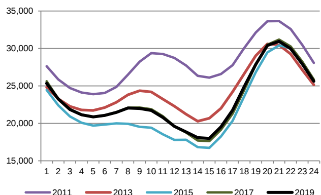
Figura 6.28 – Domanda residua media oraria nei giorni festivi
