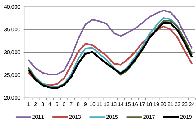
Figura 6.27 – Domanda media oraria totale e residua nel 2019
